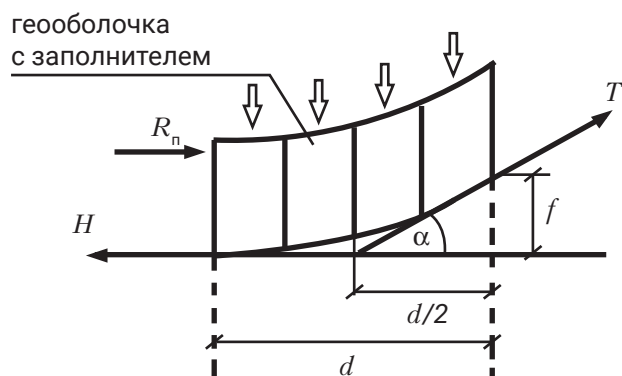
Рис. 4. Фрагмент вырезанной части геоболочки
