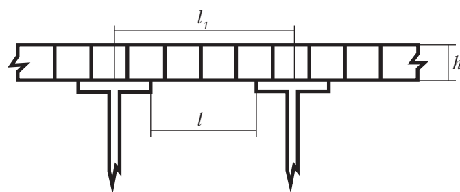
Рис. 2. Схема ростверка, сооруженного с применением геоболочки
