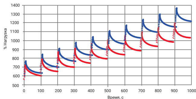
Рис. 4. Увеличение плотности фазы СБС-полимера в битуме улучшает релаксационные способности вяжущего
