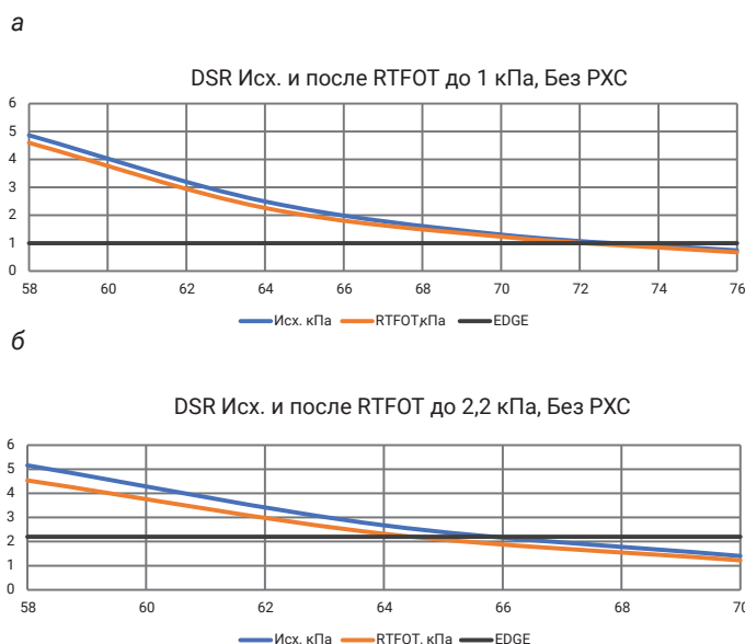
Рис. 1. Изменения вязкости составов до и после RTFOT: а — с устойчивостью не менее 1 кПа; б — с устойчивостью не менее 2,2 кПа (без регулируемой химической стабилизации, РХС)
