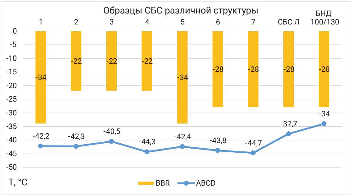
Рис 1. Сравнительная оценка нижнего температурного предела по PG ПБВ, модифицированных различными образцами СБС, по методикам BBR и ABCD
