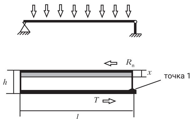
Рис. 3. Расчетная схема балки (геооболочки)
