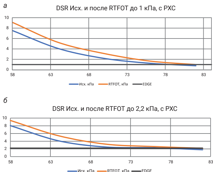
Рис. 2. Изменения вязкости составов до и после RTFOT: а — с устойчивостью не менее 1 кПа; б — с устойчивостью не менее 2,2 кПа (с регулируемой химической стабилизацией, РХС)
