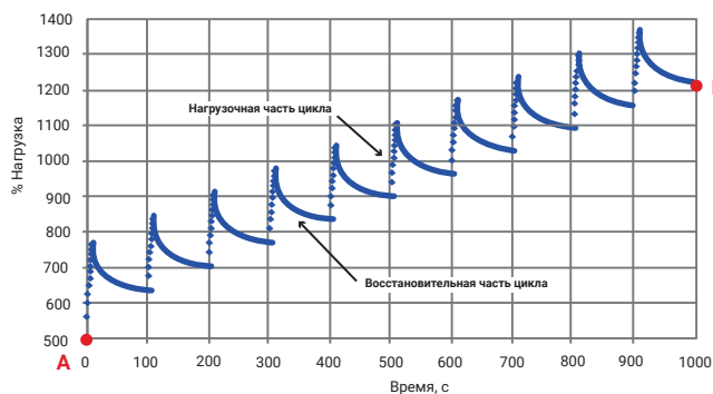
Рис. 3. Накопленная деформация после многократного нагружения релаксации, разница в % между точками А и Б
